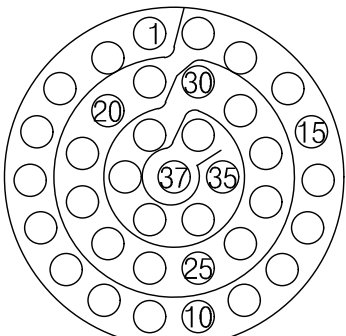
YH38999/46WD35PN 연결기 후면도 #22D-37EA
