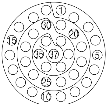
YH38999/24WD35SN 연결기 후면도 #22D-37EA
