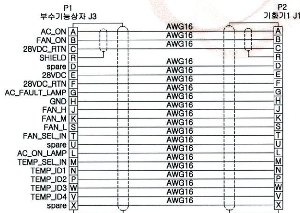
배선도
