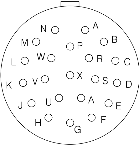
YH3474L22-21SN 연결기 후면도 #16-21EA
