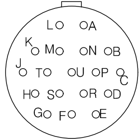
YH3474L14-18SN 연결기 후면도 #20-18EA
