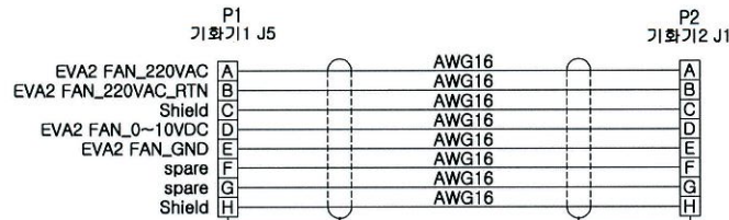
배선도
