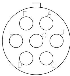
YHB030-16S-1P 연결기 후면도 #16-7EA
