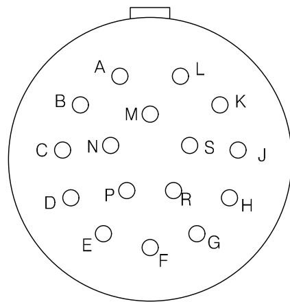
YH3474L20-16PN 연결기 후면도 #16-16EA
