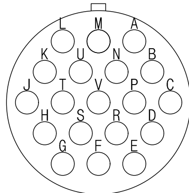
YH3100A22-14SN 연결기 후면도 #16-19EA
