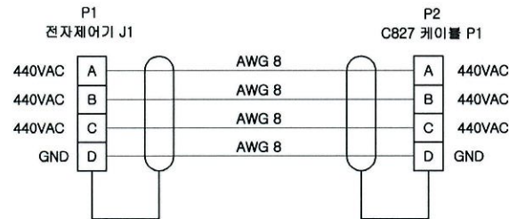
배선도
