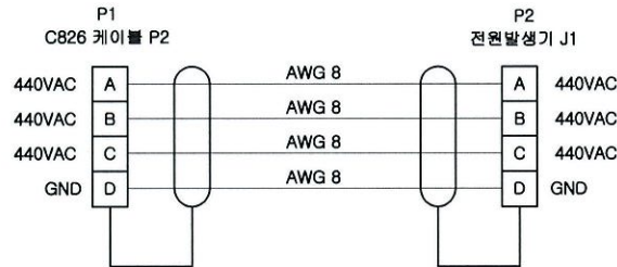
배선도
