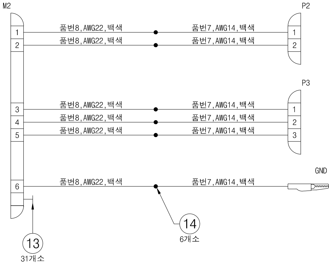
배선도
