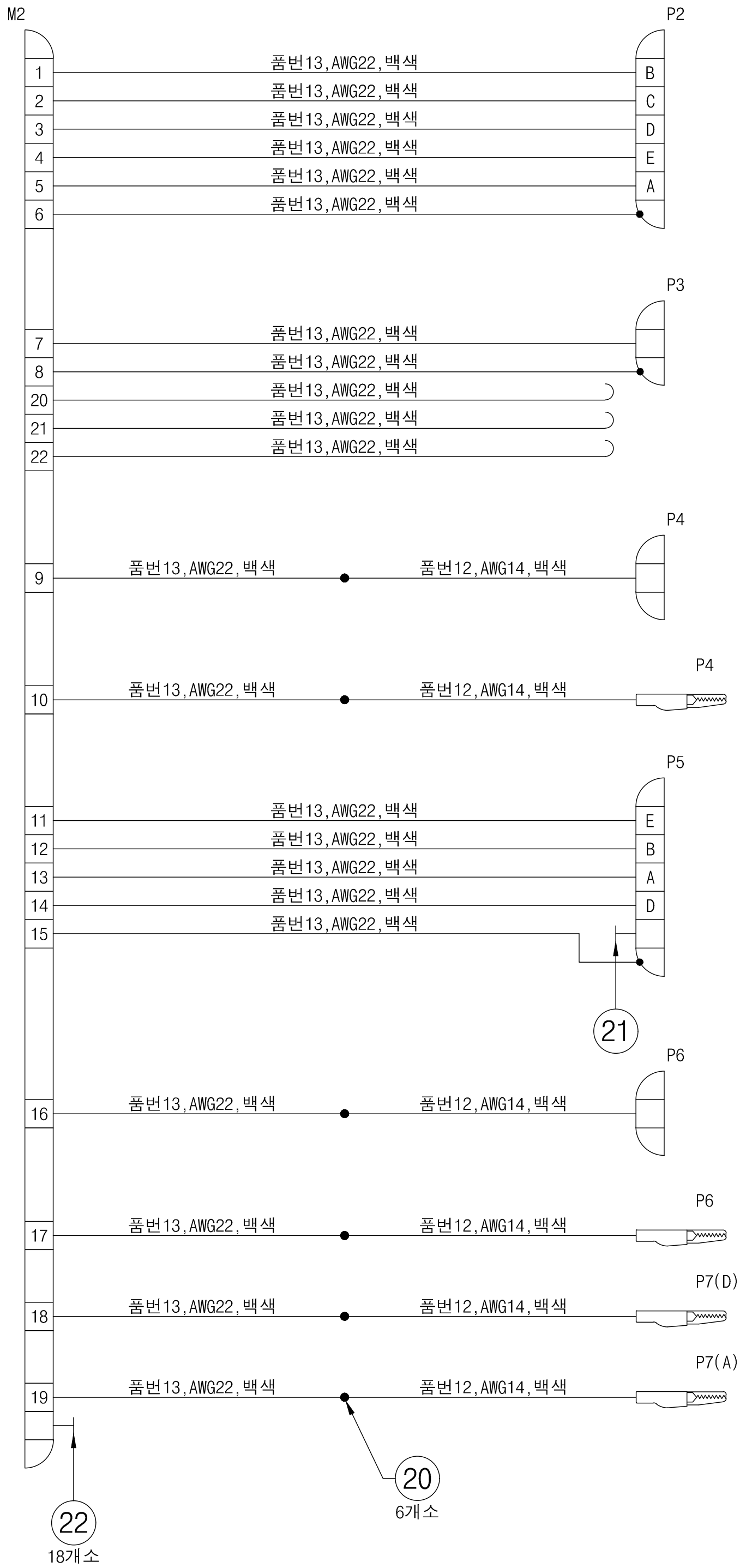
배선도
