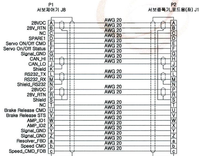
배선도
