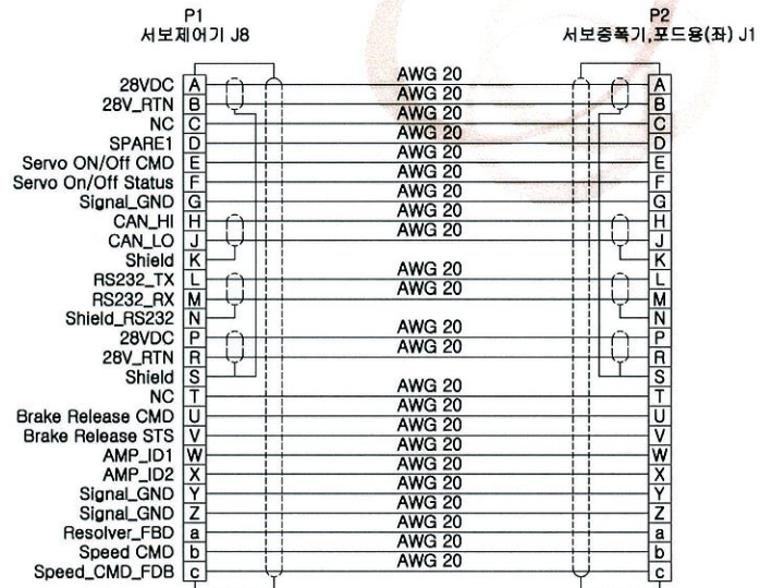
배선도
