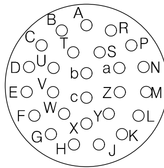
YH38999/44FE26PN 연결기 후면도 #20-26EA
