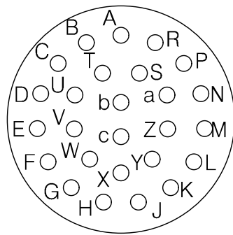
YH38999/44FE26PN 연결기 후면도 #20-26EA
