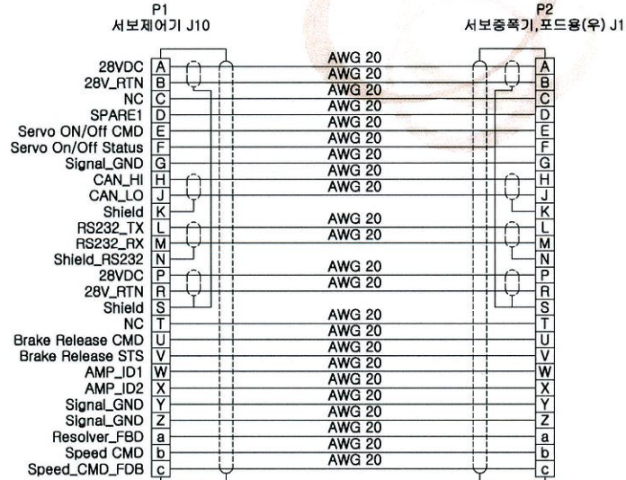
배선도
