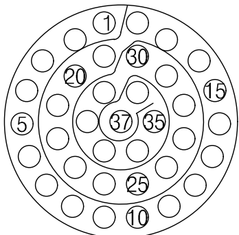
연결기 후면도 #22D-37EA
