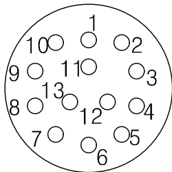
연결기 후면도 #22D-13EA
