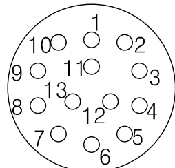
YH38999/44FB35SN 연결기 후면도 #22D-13EA
