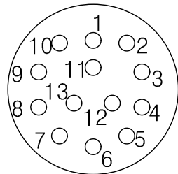
YH38999/44FB35SN 연결기 후면도 #22D-13EA
