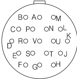
YH3474L14-19P 연결기 후면도 #20-19EA
