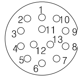
YH38999/24FB35PN 연결기 후면도 #22D-13EA
