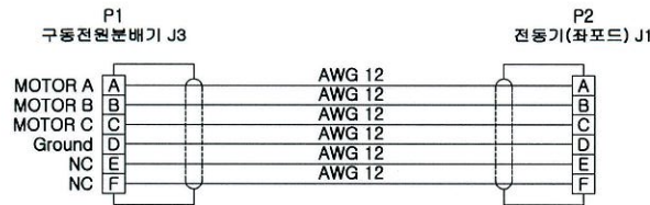
배선도
