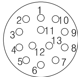
YH38999/44FB35PN 연결기 후면도 #22D-13EA
