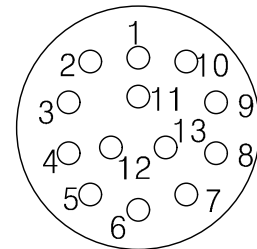
YH38999/24FB35PN 연결기 후면도 #22D-13EA
