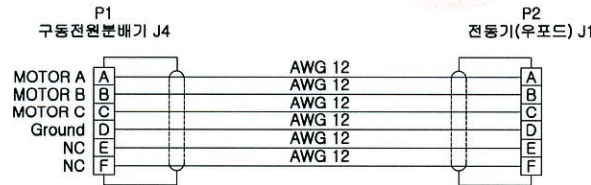
배선도
