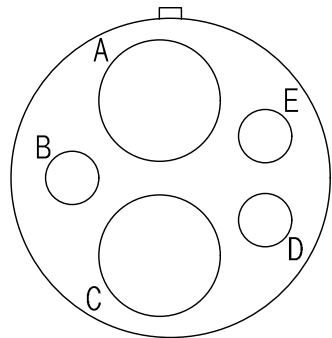
YHB030-24-12P 연결기 후면도 #8-2EA #16-3EA
