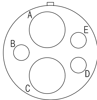
YHB030-24-12P 연결기 후면도 #8-2EA #16-3EA
