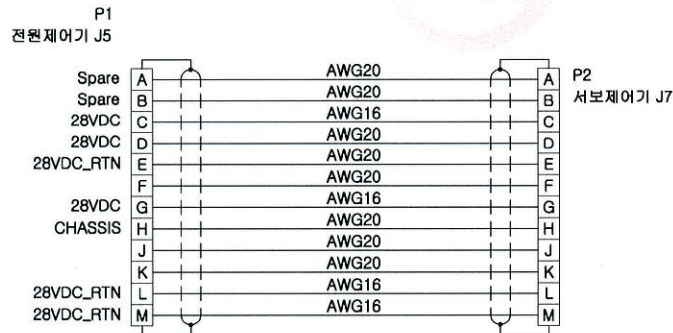
배선도
