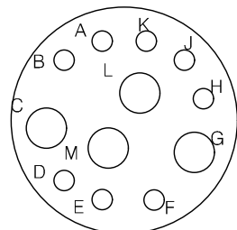
YH38999/44WD97PN 연결기 후면도 #16-4EA #20-8EA
