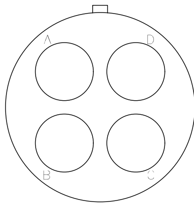
MS17347R22C22P 연결기 후면도 #8-4EA
