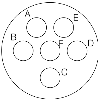
YH38999/44WE6PN 연결기 후면도 #12-6EA
