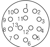
YH38999/44WB35SN 연결기 후면도 #22D-13EA
