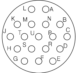
YH38999/44WD18SN 연결기 후면도 #20-18EA
