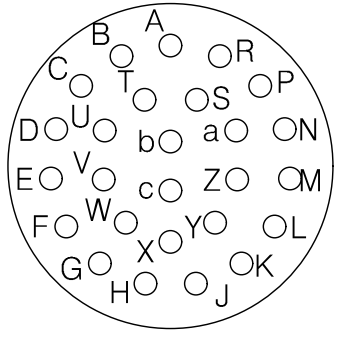
YH38999/44WE26PN 연결기 후면도 #20-26EA
