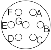
YH38999/46WB99SN 연결기 후면도 #20-7EA
