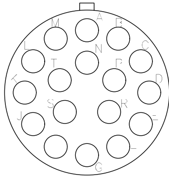
YHB030-20-29S 연결기 후면도 #16-17EA
