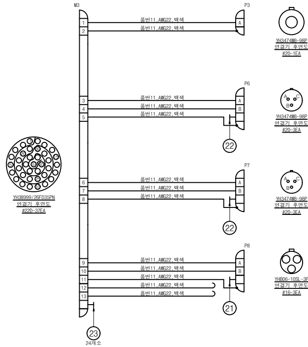
배선도
