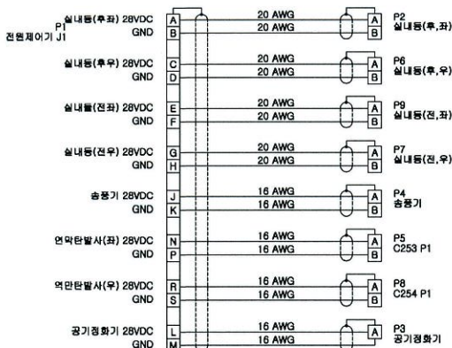
배선도
