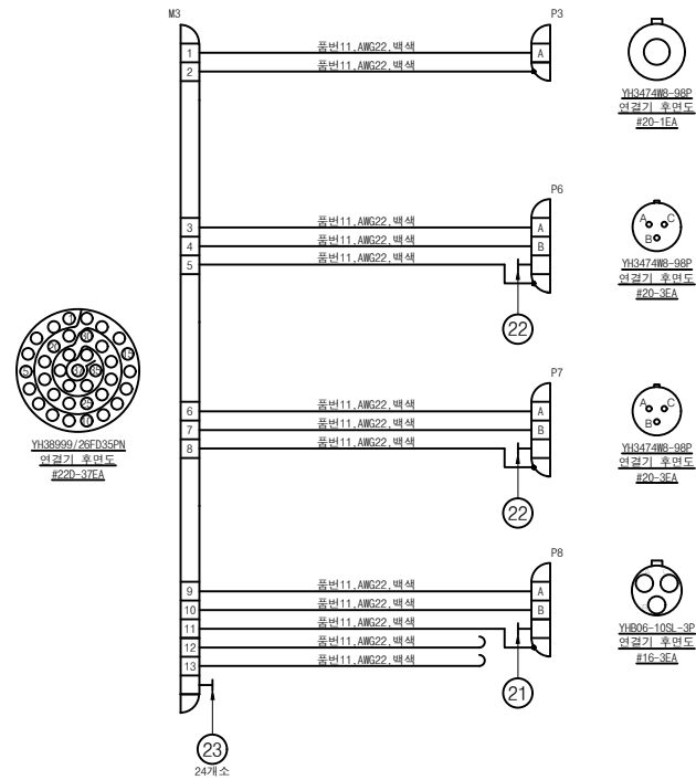
배선도
