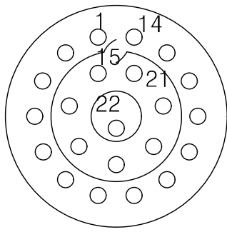
YH38999/44WC35PA 연결기 후면도 #22D-22EA
