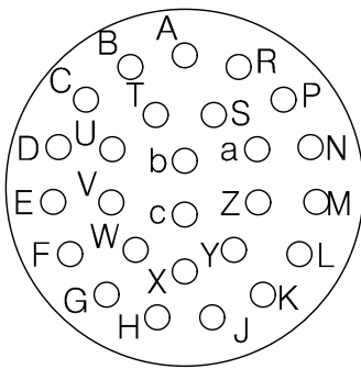
YH38999/44WE26PA 연결기 후면도 #20-26EA
