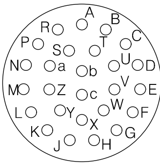
YH38999/44WE26SA 연결기 후면도 #20-26EA
