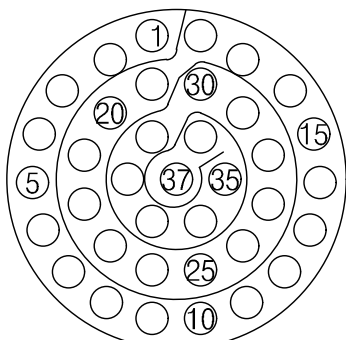
YH38999/26FD35PN 연결기 후면도 #22D-37EA
