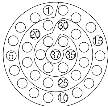
YH38999/26FD35PN 연결기 후면도 #22D-37EA
