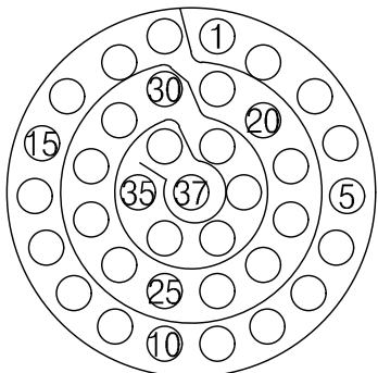
YH38999/24WD35SN 연결기 후면도 #22D-37EA
