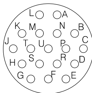
YH38999/44WD18SN 연결기 후면도 #20-18EA
