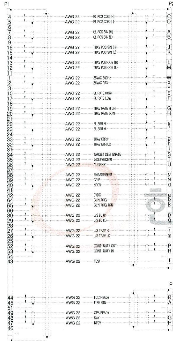
케이블 결선도
