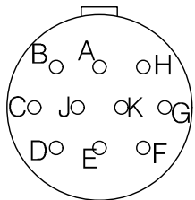
YH3474W12-10PN 연결기 후면도 #20-10EA
