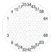
D38999/46WF35SA 연결기 후면 투영도 #22D-66EA
