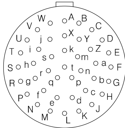
YH3474W20-41SW 연결기 후면도 #20-41EA
