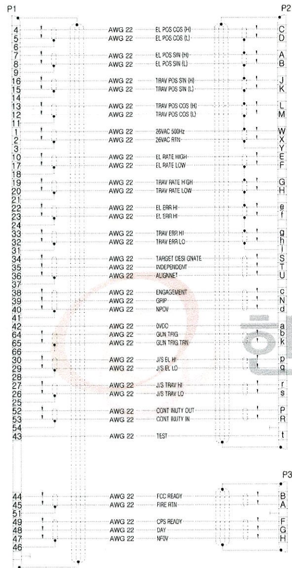
케이블 결선도
