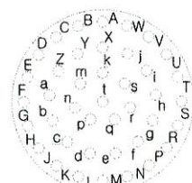
MS3475W20-41PW 연결기 후면 투영도 #20-41EA
