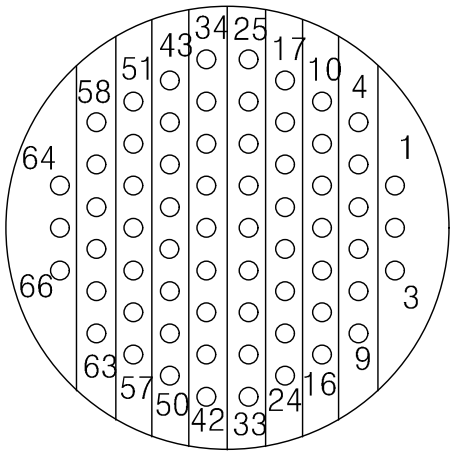
YH38999/44WF35PA 연결기 후면도 #22D-66EA
