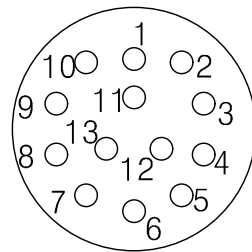
YH38999/44WB35SA 연결기 후면도 #22D-13EA
