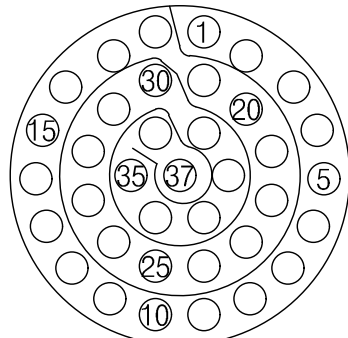
YH38999/44WD35SN 연결기 후면도 #22D-37EA
