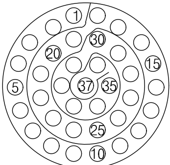
YH38999/44WD35PN 연결기 후면도 #22D-37EA
