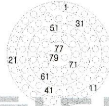
D38999/46WG35SN 연결기 후면 투영도 #22D-79EA
