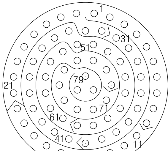
YH38999/44WG35SN 연결기 후면도 #22D-79EA
