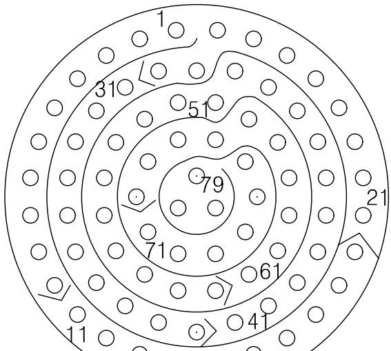
YH38999/44WG35PN 연결기 후면도 #22D-79EA
