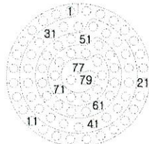
D38999/46WG35PN 연결기 후면 투영도 #22D-79EA
