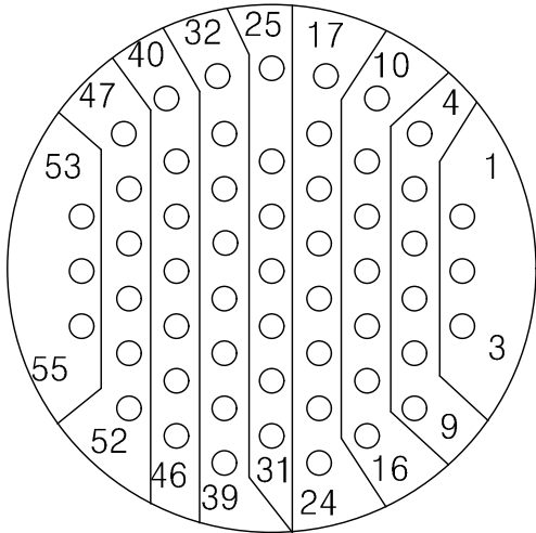
SJT07RT16-35PN 연결기 후면도 #22D-55EA
