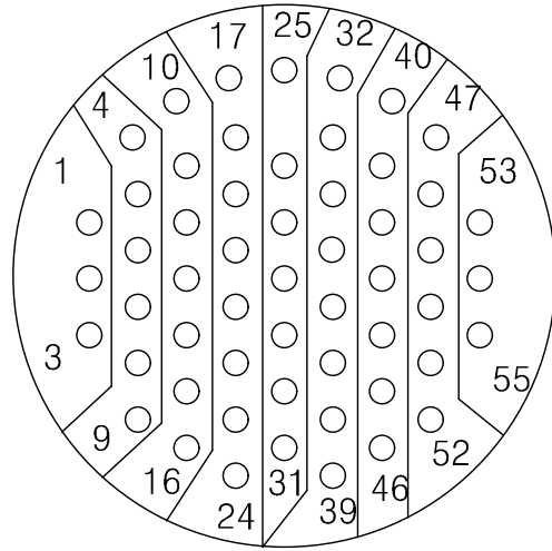
YH38999/44WE35SN 연결기 후면도 #22D-55EA
