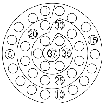
YH38999/44WD35PN 연결기 후면도 #22D-37EA
