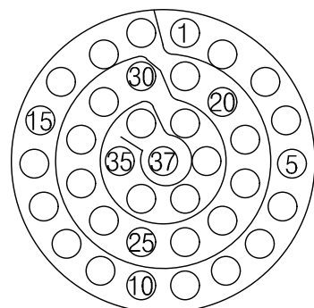
YH38999/44WD35SN 연결기 후면도 #22D-37EA
