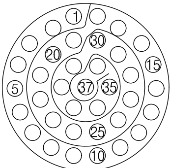
YH38999/44WD35PB 연결기 후면도 #22D-37EA
