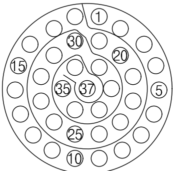
YH38999/44WD35SB 연결기 후면도 #22D-37EA
