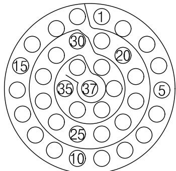
YH38999/44WD35SB 연결기 후면도 #22D-37EA
