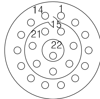
YH38999/44WC35SA 연결기 후면도 #22D-22EA
