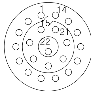
YH38999/44WC35PA 연결기 후면도 #22D-22EA
