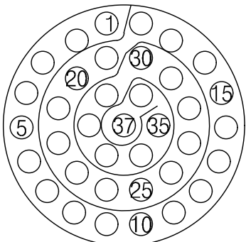
YH38999/44WD35PD 연결기 후면도 #22D-37EA
