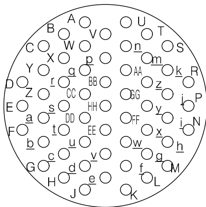
YH38999/44WH55PA 연결기 후면도 #20-55EA
