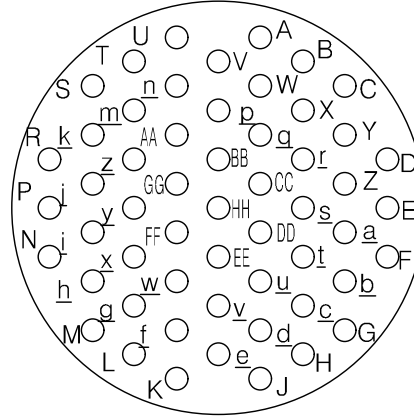
YH38999/44WH55SN 연결기 후면도 #20-55EA
